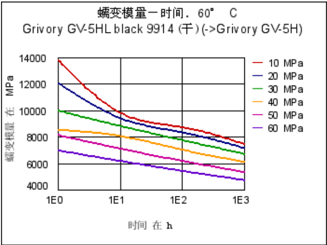
蠕变模量 - 时间. 60 °C
